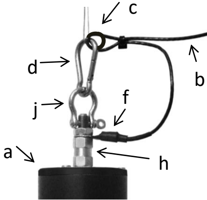
Plate 5. Hybrid Micro / Mini Connections.
