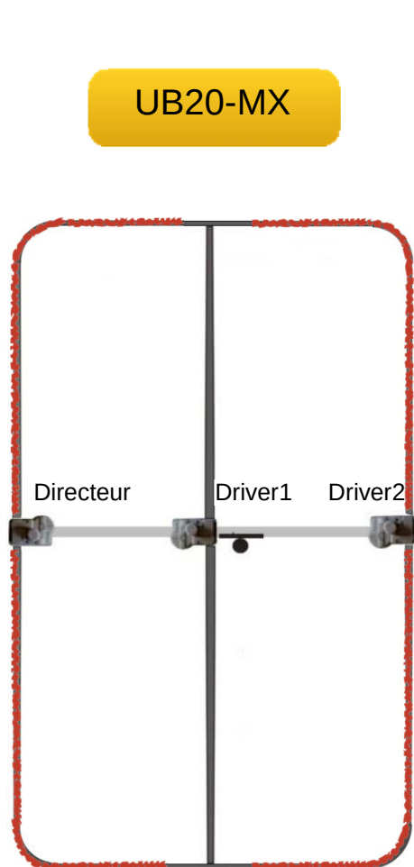
2 éléments Moxon lorsque l'on est en 20 mètres
