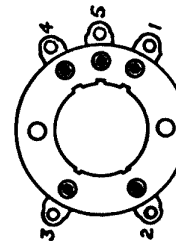
SAA & 7AA (ACORN VALVES)
