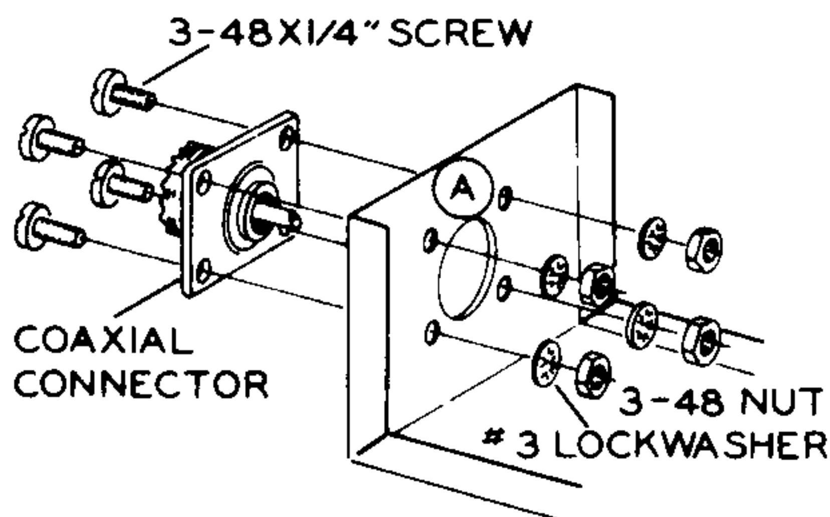
Detail 1A
