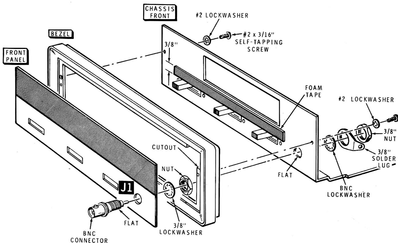
Detail 4-1E
