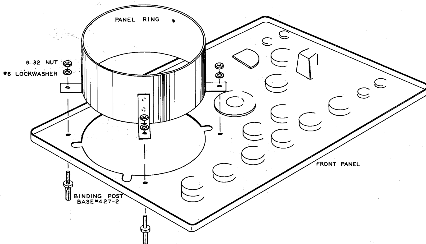
Detail 1E
