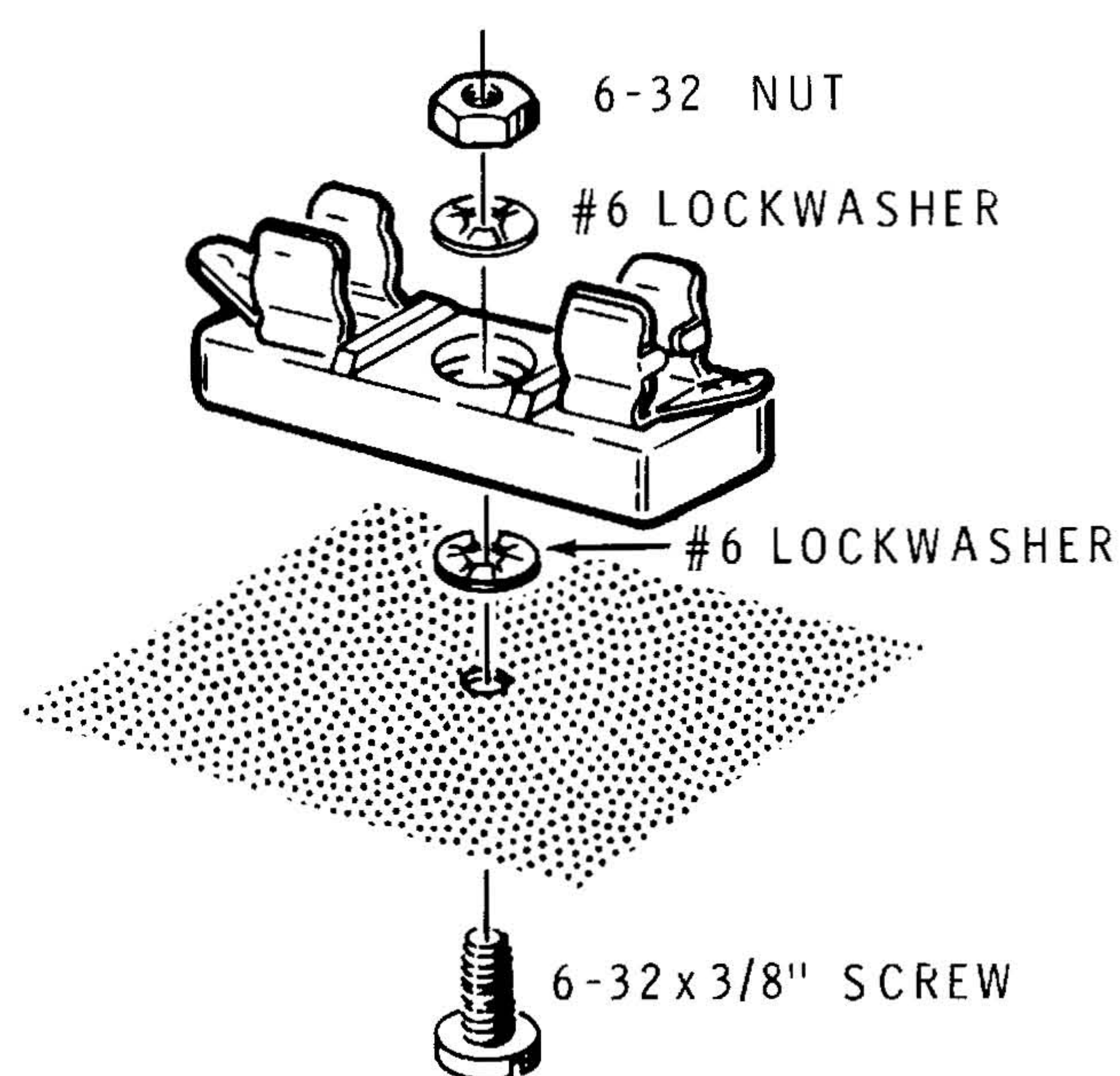
Detail 2-2E
