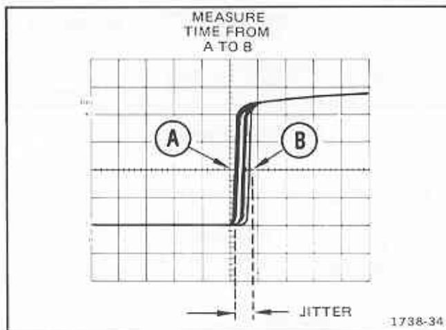
Fig. 23. Pulse jitter.
