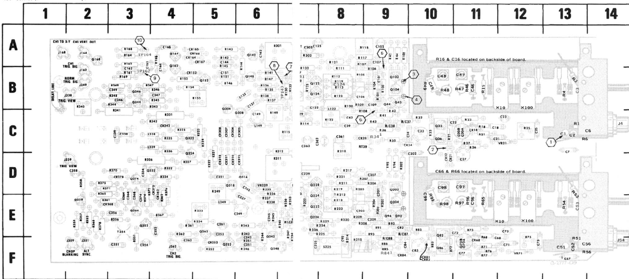
Fig. 8-2. A1 &amp; A2—Attenuators
