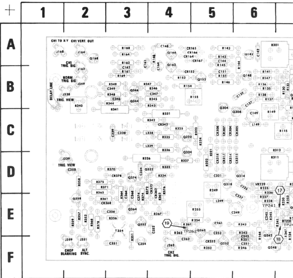
Fig. 8-4. A1 &amp; A2—Atb
