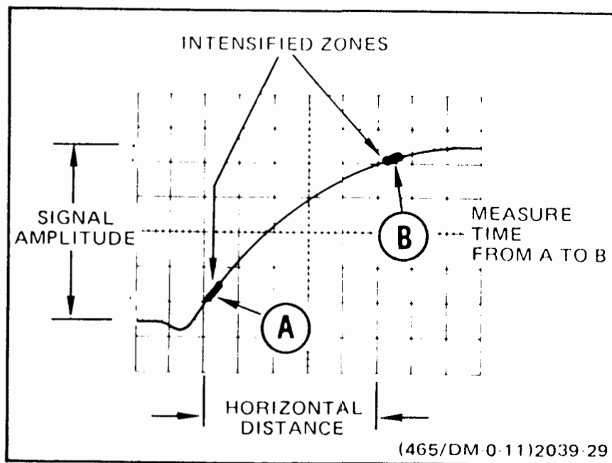
Fig. 28. Risetime.
