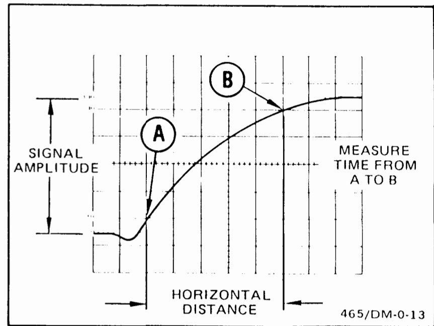
Fig. 19. Risetime.
