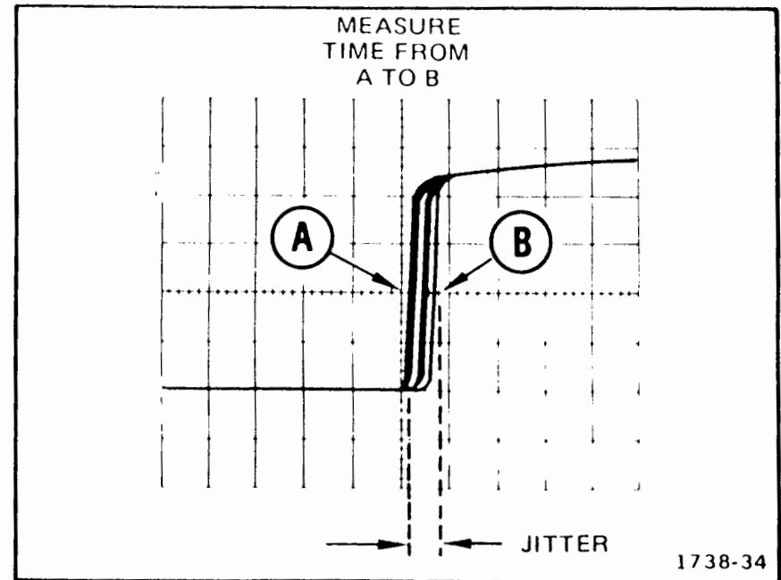
Fig. 23. Pulse jitter.
