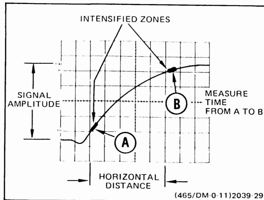
Fig. 32. Risetime.
