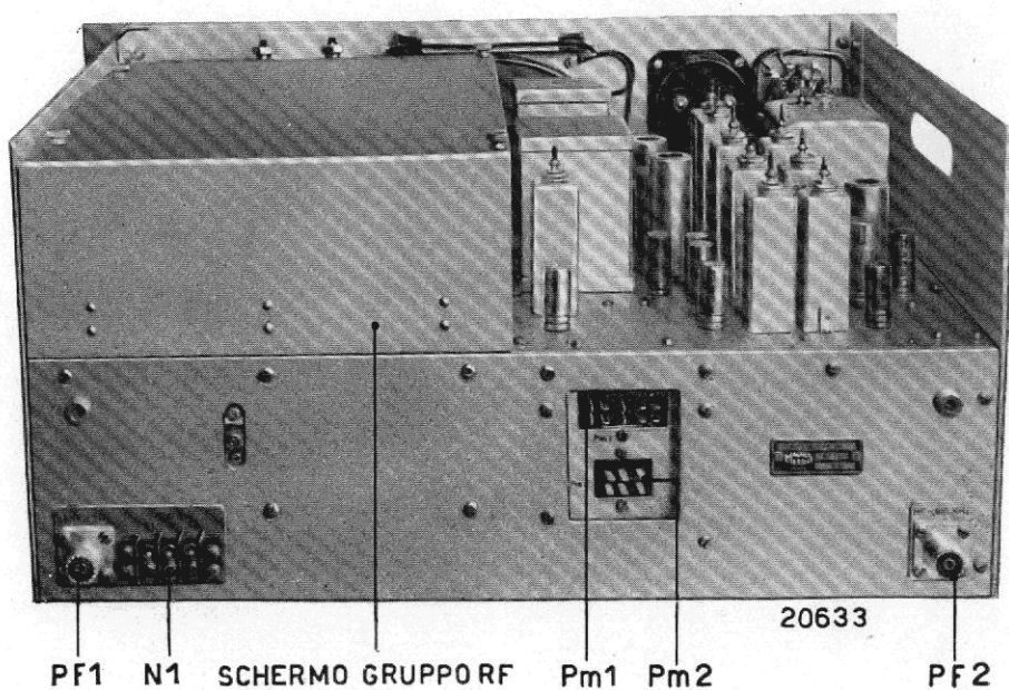
71.4 - Telaio completo RP 32 - Vista posteriore con prese di collegamento
