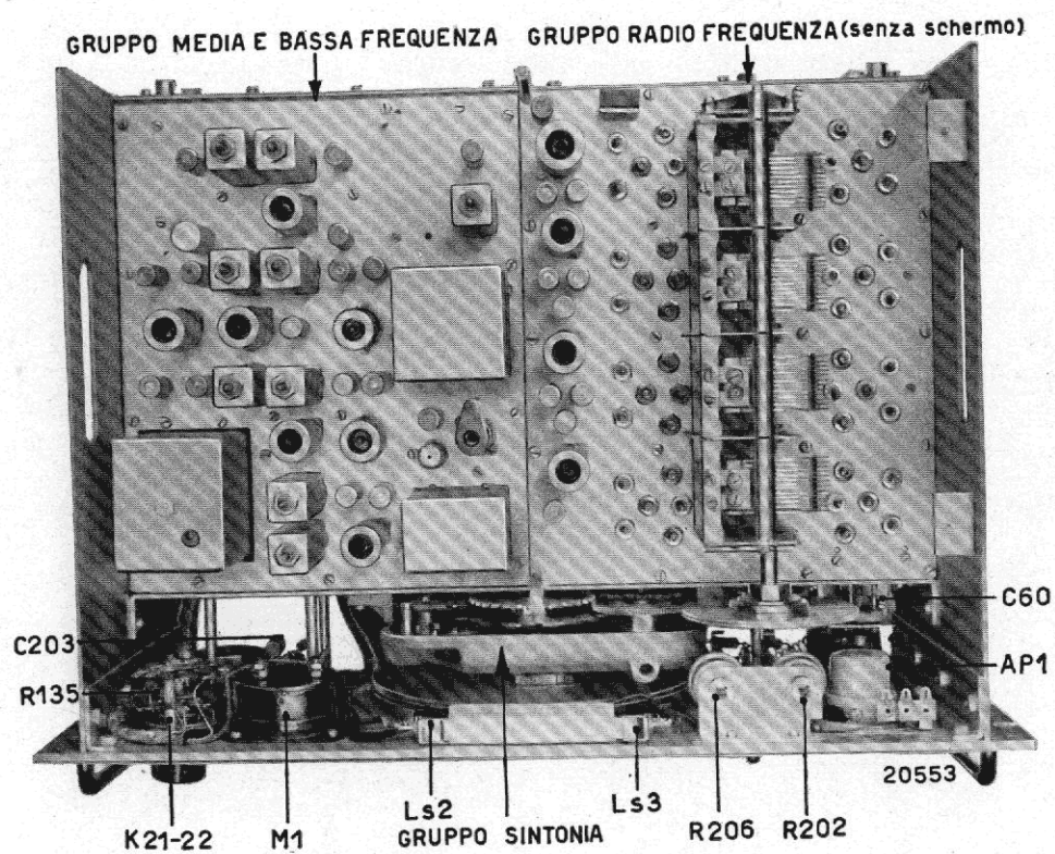
72.1 - Telaio completo RP 32 - Vista superiore
