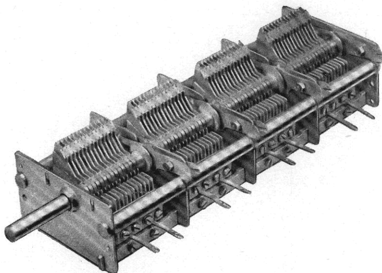
74.5 - Condensatore variabile multiplo
