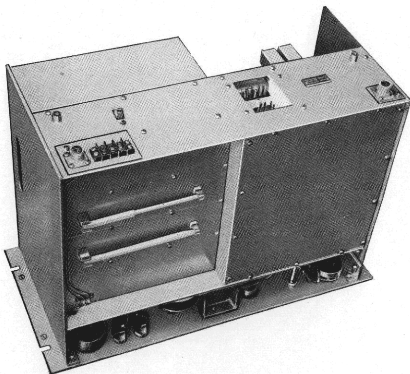
71.2 - Telaio completo RP 32 - Vista inferiore, con schermi e giraviti
