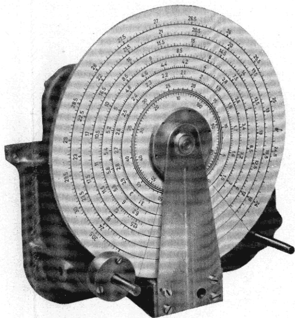
74.3 - Gruppo Sintonia - Scala
