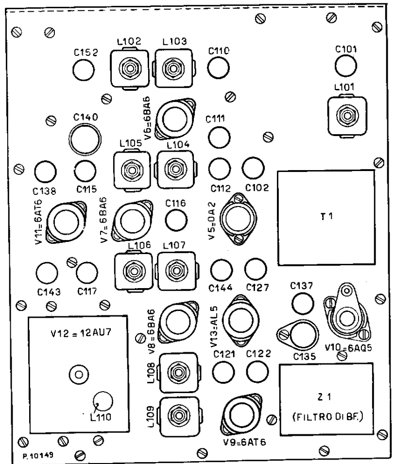
72.2 - Gruppo MF - BF - Vista superiore
