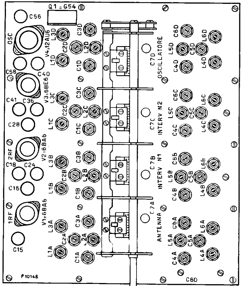
72.3 - Gruppo RF - Vista superiore
