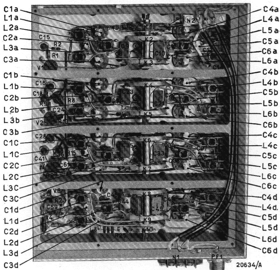
73.3 - Gruppo RF - Vista inferiore
