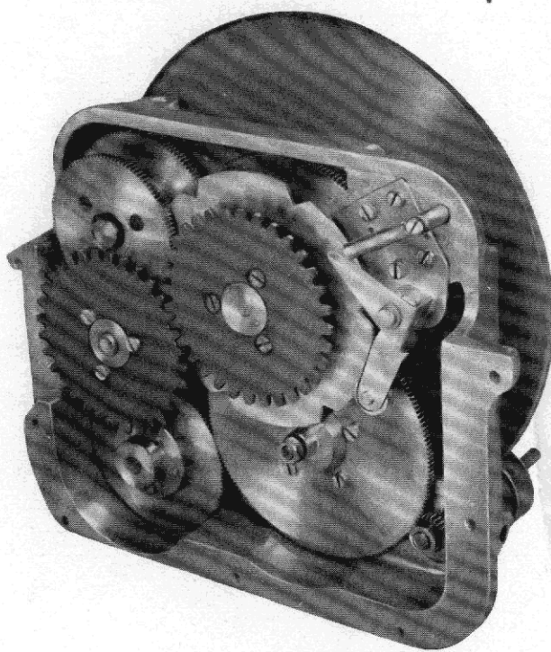
74.4 - Gruppo Sintonia - Domoltiplica
