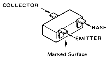
2SA812 (M4) (Q403)
