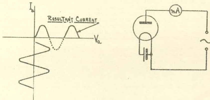
FIG. 17C.—Diode rectification.
