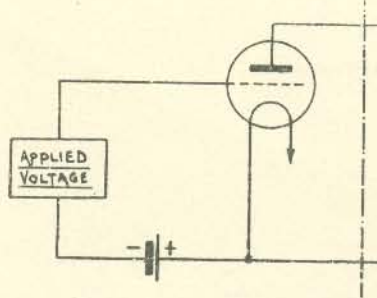
FIG. 18. Battery bias.
