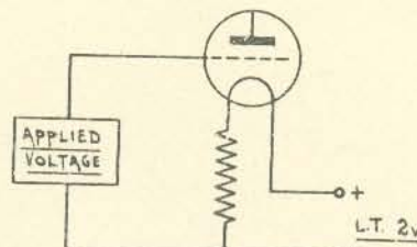
FIG. 19. Filament bias.
