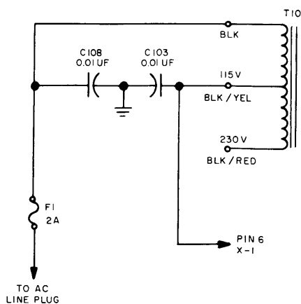
115 VOLT OPERATION
