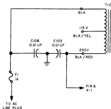
230 VOLT OPERATION
