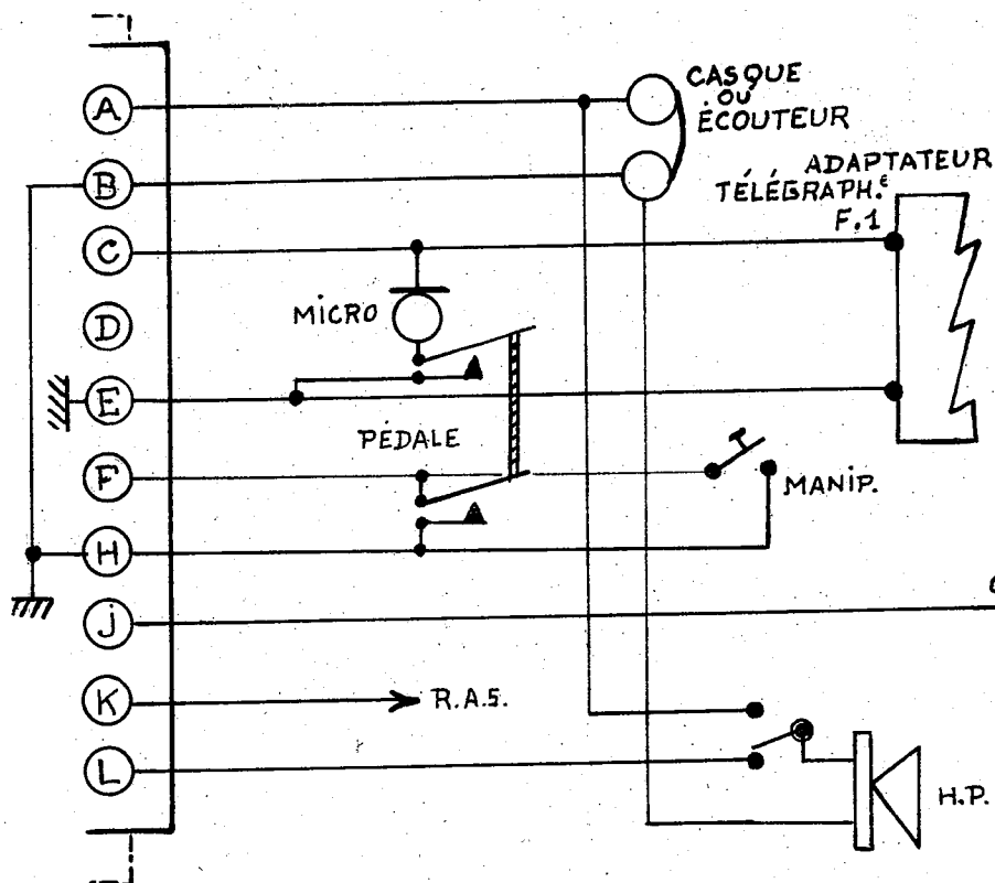
CASQUE H 63/U
