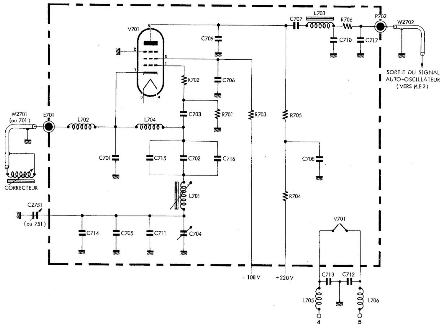
Fig. 13 AUTO-OSCILLATEUR
