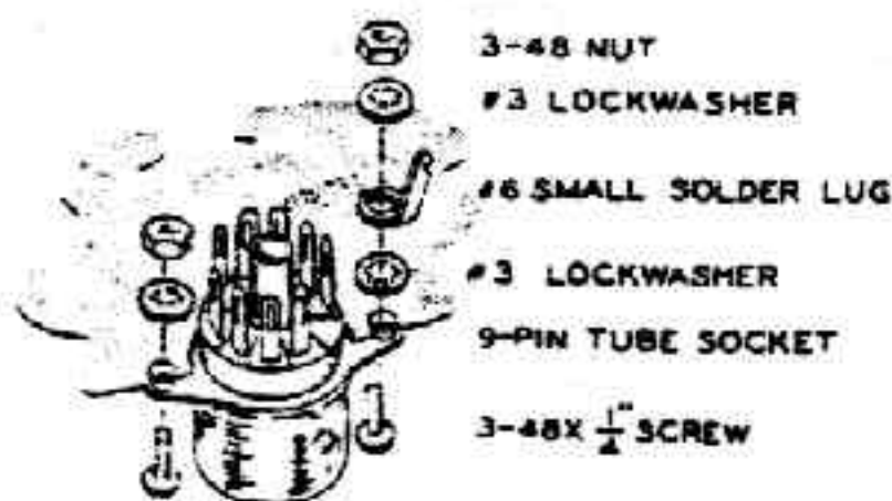
Detail 1A
