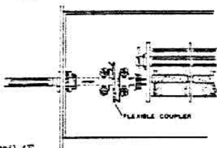
Detail 4E
