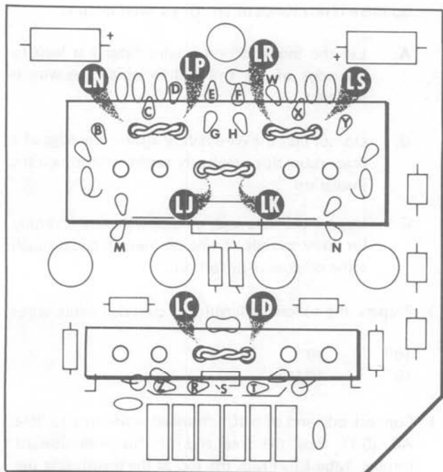
Detail 11-5E
