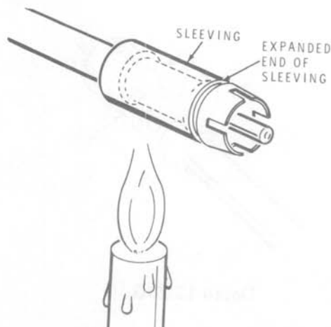
Detail 12-28E
