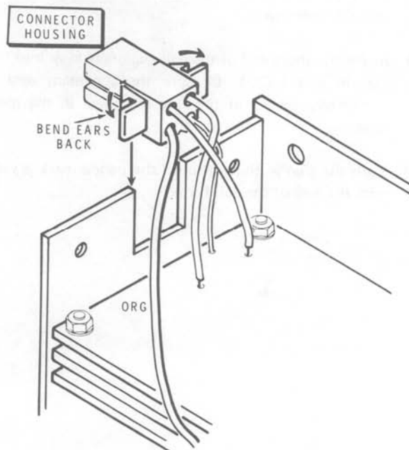
Detail 1-12E
