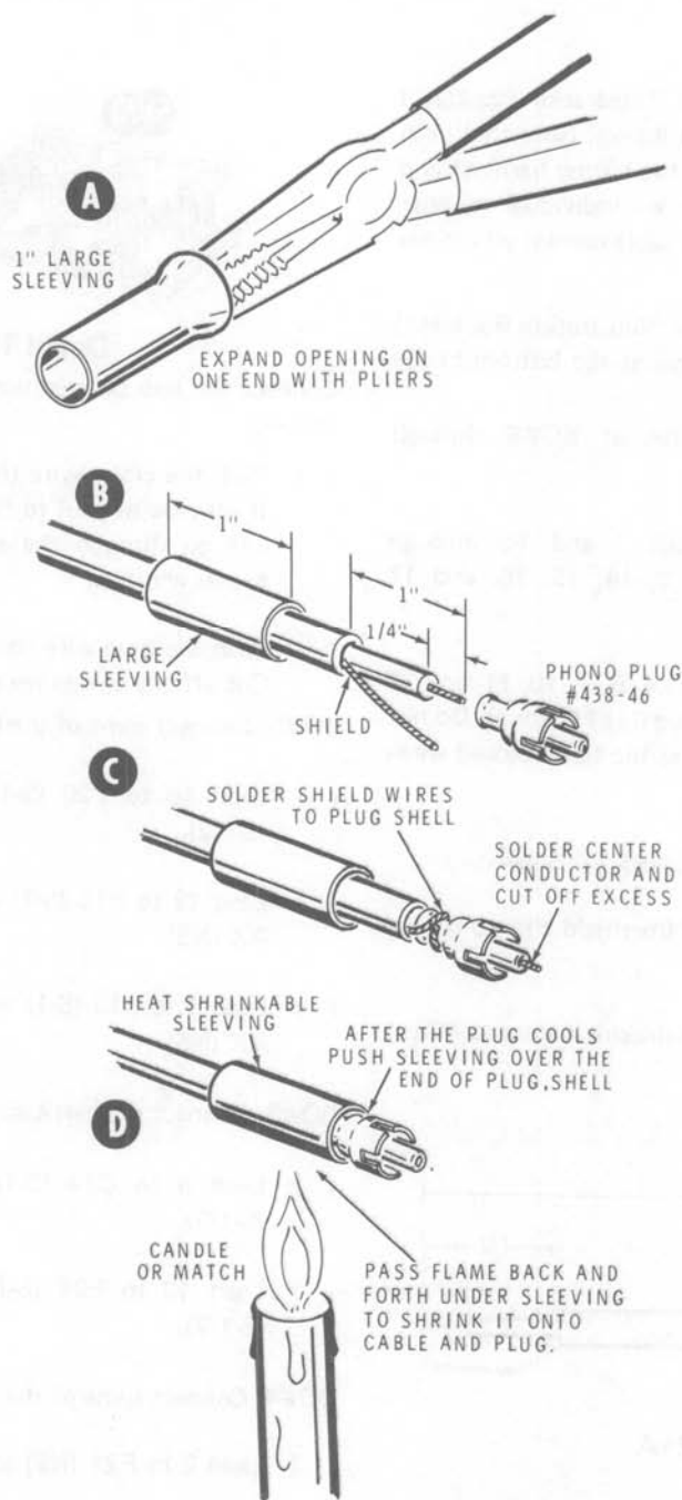
Detail 12-19E
