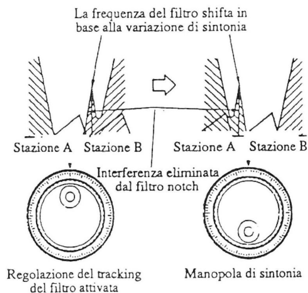
Figura 6.4 - Intervento del filtro notch
