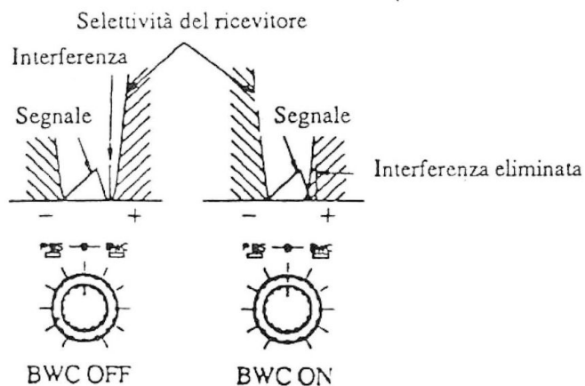
Figura 6.2 - Controllo dell'ampiezza della banda passante
