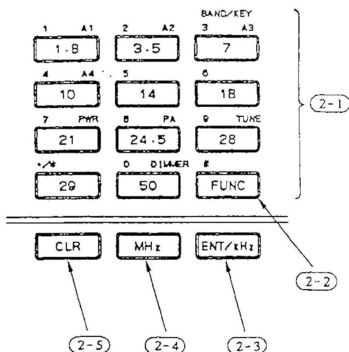
Figura 4.3 - La tastiera numerica
