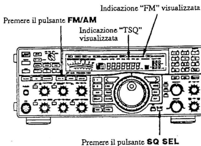
Figura 6.10 - Uso del tone squelch
