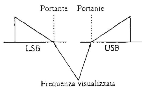
Figura 5.2 - Frequenza visualizzata in modo SSB
