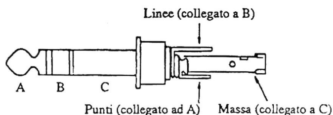
Figura 6.13 - Collegamento di un tasto CW
