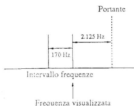
Figura 5.5 - Visualizzazione della frequenza in AFSK
