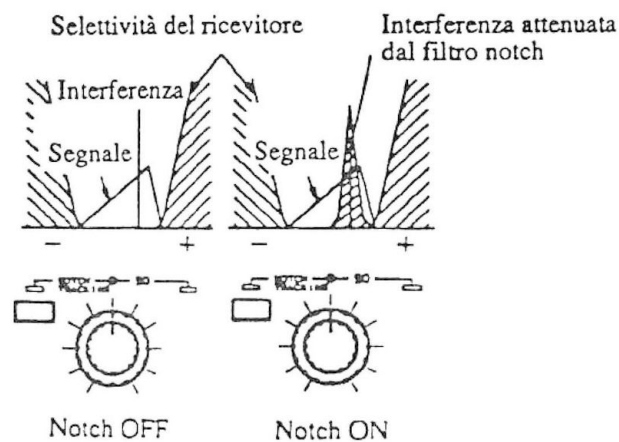
Figura 6.3 - Intervento del filtro notch
