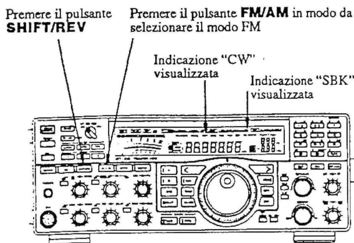
Figura 6.9 - Shift frequenze per aggancio a ripetitore
