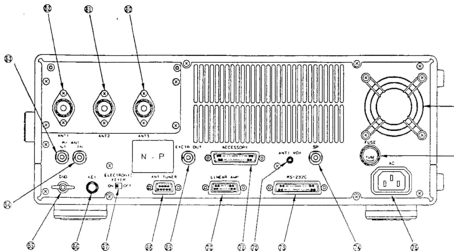
Figura 4.3 - Il pannello posteriore
