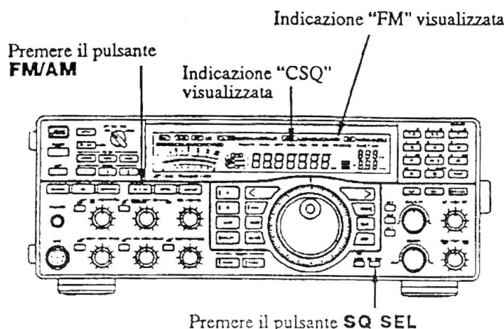
Figura 6.11 - Uso del code squelch
