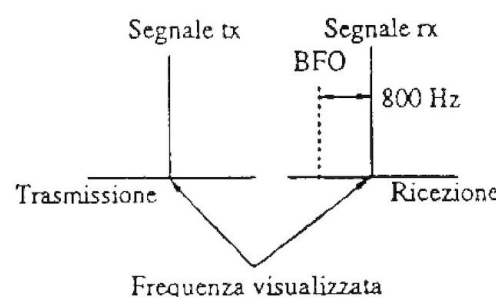
Figura 5.3 - Visualizzazione della frequenza in CW
