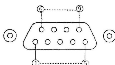
Figura 4.7 - Piedinatura del connettore per accordatore d'antenna (vista dall'esterno del pannello posteriore)
