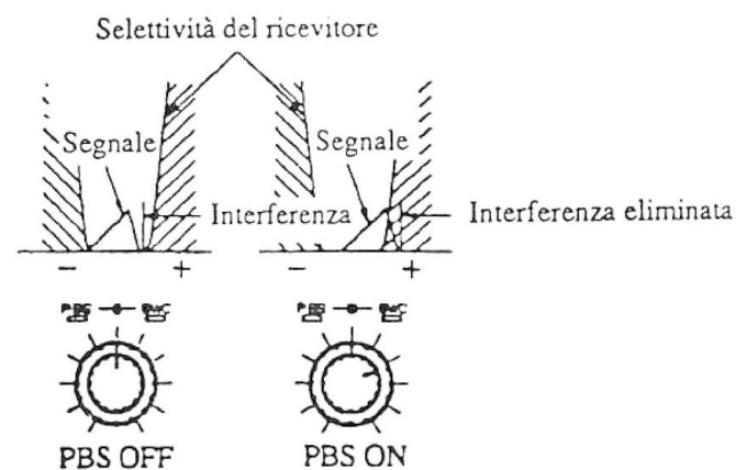
Figura 6.1 - Scostamento della banda passante
