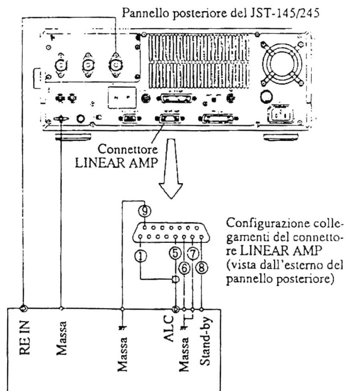
Figura 6.14 - Collegamento di un amplificatore lineare
