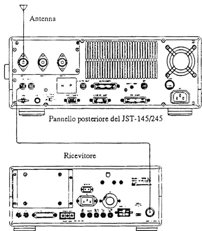
Figura 6.16 - Collegamento di un ricevitore esterno
