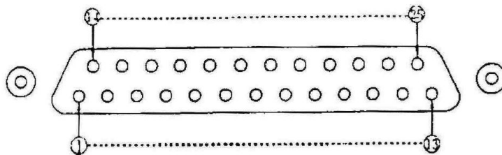
Figura 4.9 - Piedinatura del connettore per interfaccia RS-232C (vista dall'esterno del pannello posteriore)
