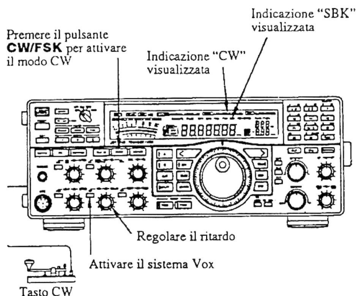
Figura 6.6 - Funzionamento in semi break-in
