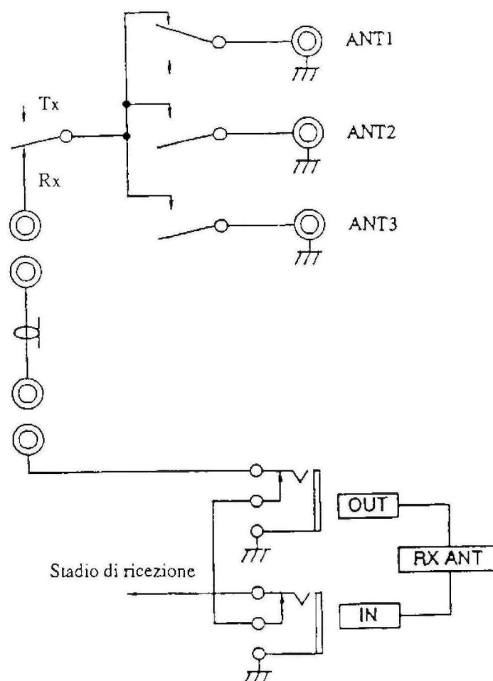
Figura 4.6 - Collegamenti interni degli ingressi antenne
