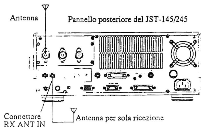
Figura 6.15 - Collegamento di un'antenna speciale
