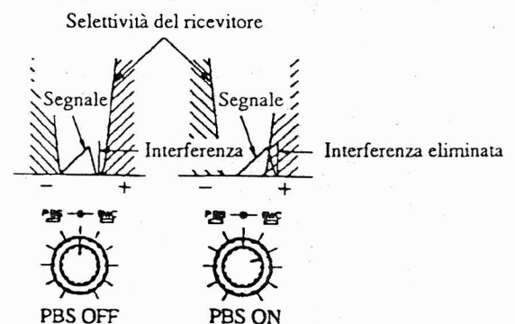
Figura 6.1 - Scostamento della banda passante
