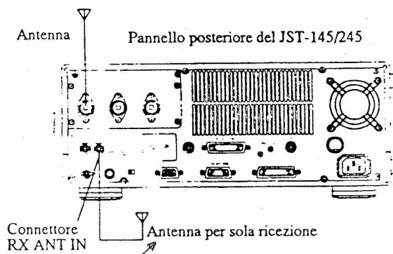
Figura 6.15 - Collegamento di un'antenna speciale
