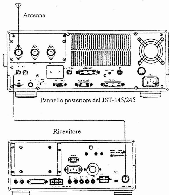
Figura 6.16 - Collegamento di un ricevitore esterno
