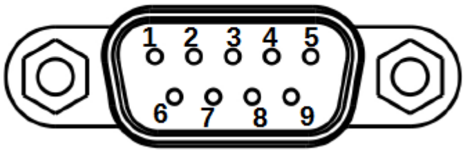
COM (Male)
