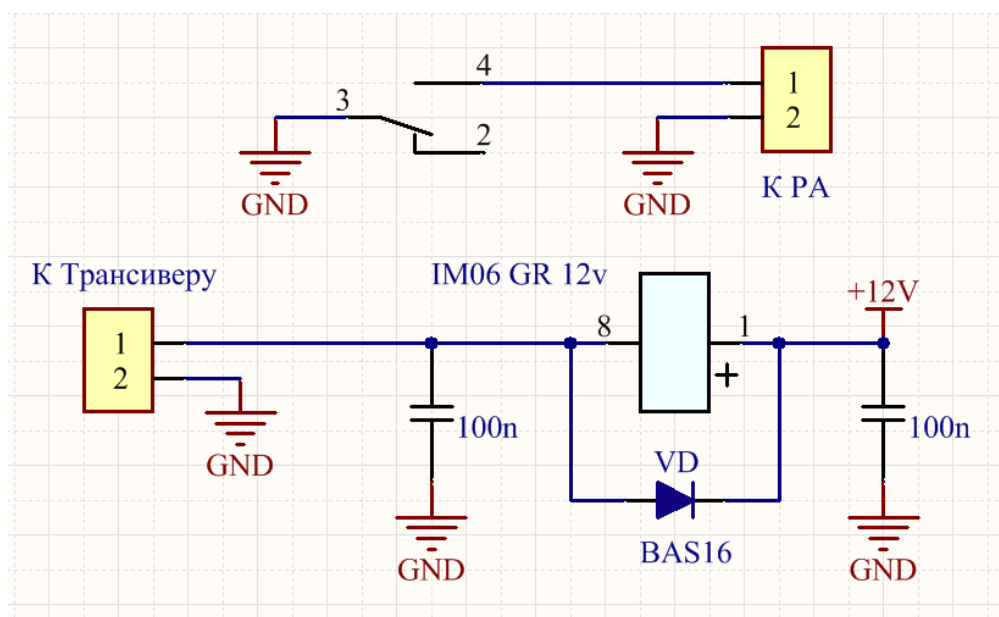
Схема коммутации.
