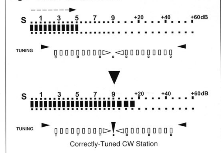
Fig. 7-4 : CW TUNING METER
