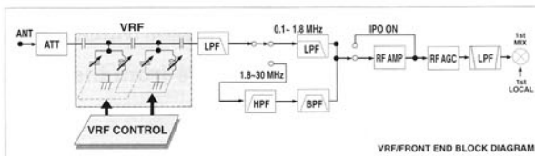
VRF/FRONT END BLOCK DIAGRAM
