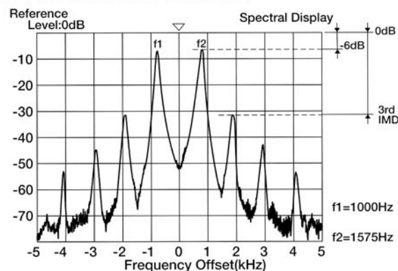
Fig. 2-7 : 2-TONE TX IMD (CLASS AB)
