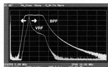
Fig.1-5 : VRF PATTERNS
