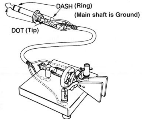
Fig. 7-6 : KEY CONNECTIONS
