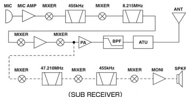
Fig. 2-3 : MONITOR CIRCUIT
