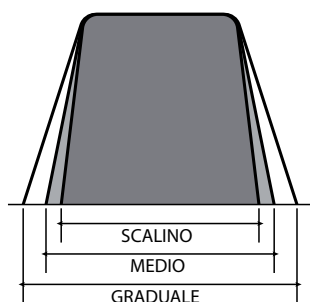
DSP BANDAPASSANTE FILTRO
