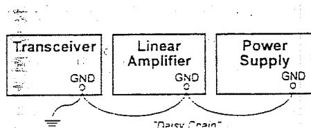
Nieprawidłowe połączenie uziemienia
