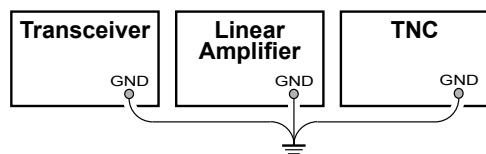
COLLEGAMENTO A TERRA CORRETTO
