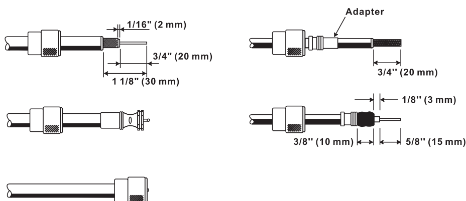
INSTALACIÓN TÍPICA PL-259
