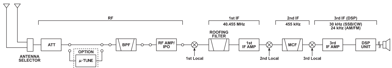
DIAGRAMA DE BLOQUES DE LA ETAPA INICIAL
