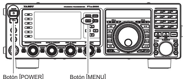
Botón [POWER]
